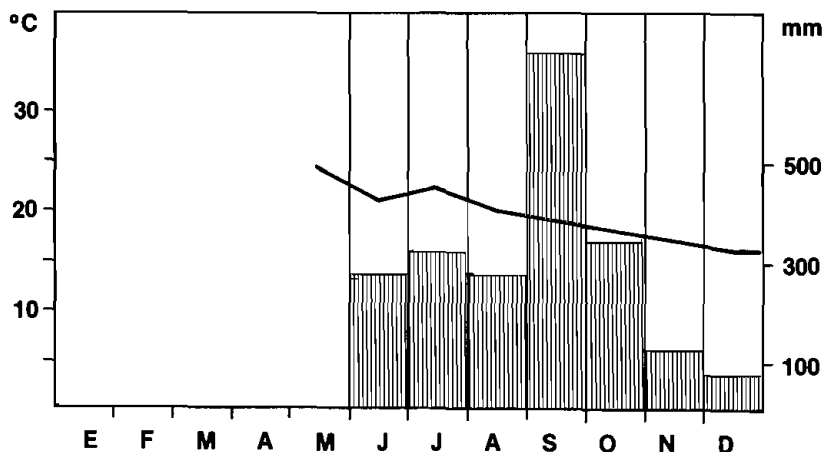
Gráfica 6 Abundancia y biomasa porcentual de los Diptera y Coleoptera necrófilos en el bosque mesófilo de Tlanchinol (1550 m), en relación con la temperatura y precipitación local. (Biomasa ilustrada con barras).
