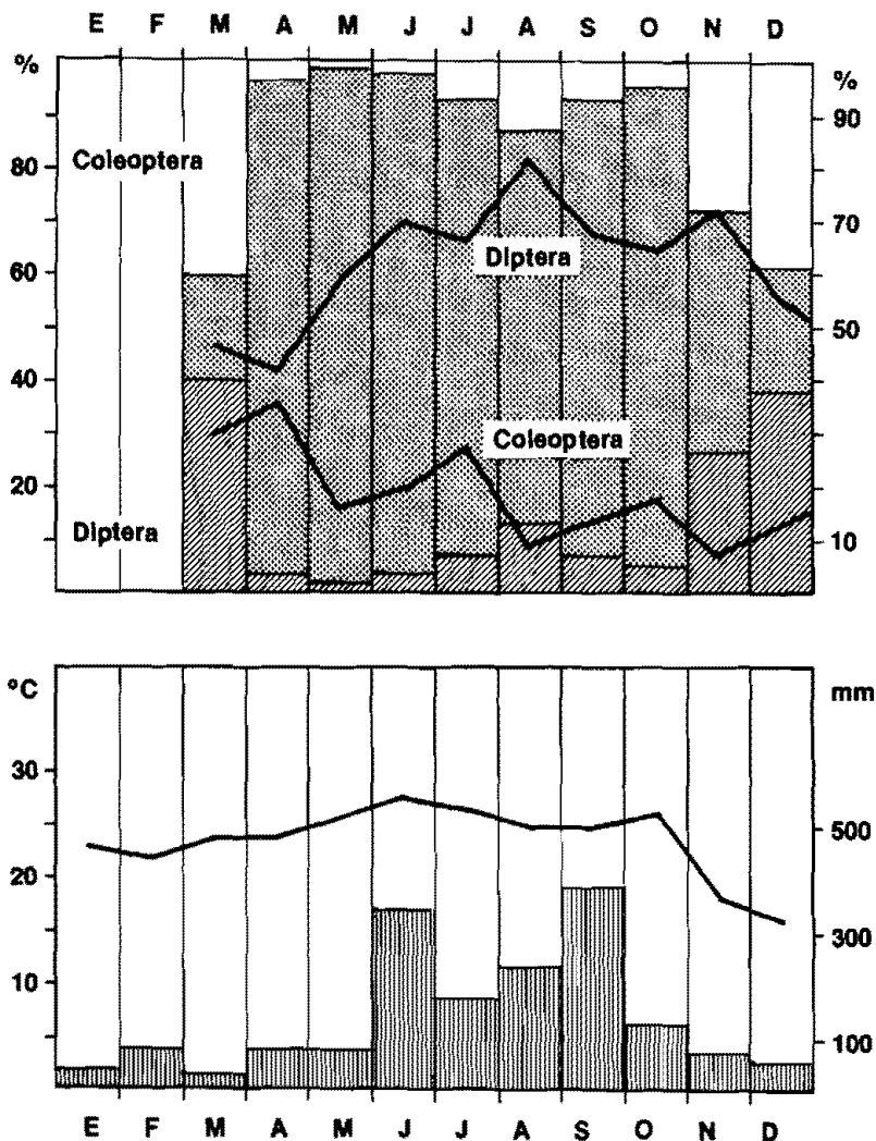
Gráfica 5 Abundancia y biomasa porcentual de los Diptera y Coleoptera necrófilos a lo largo de un año en el bosque mesófilo de Otongo (1120 m), en relación con la temperatura y precipitación local. (Biomasa ilustrada con barras).
